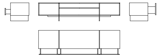
ML312 L2200 X H430 X P500MM BASE TV PARA ESTANTE MILLER C/ MÓDULO PARA BOX E PÉ EM METAL MEUBLE TV MILLER AVEC PIEDS EN MÉTAL MILLER TV CHEST WITH METAL LEGS
